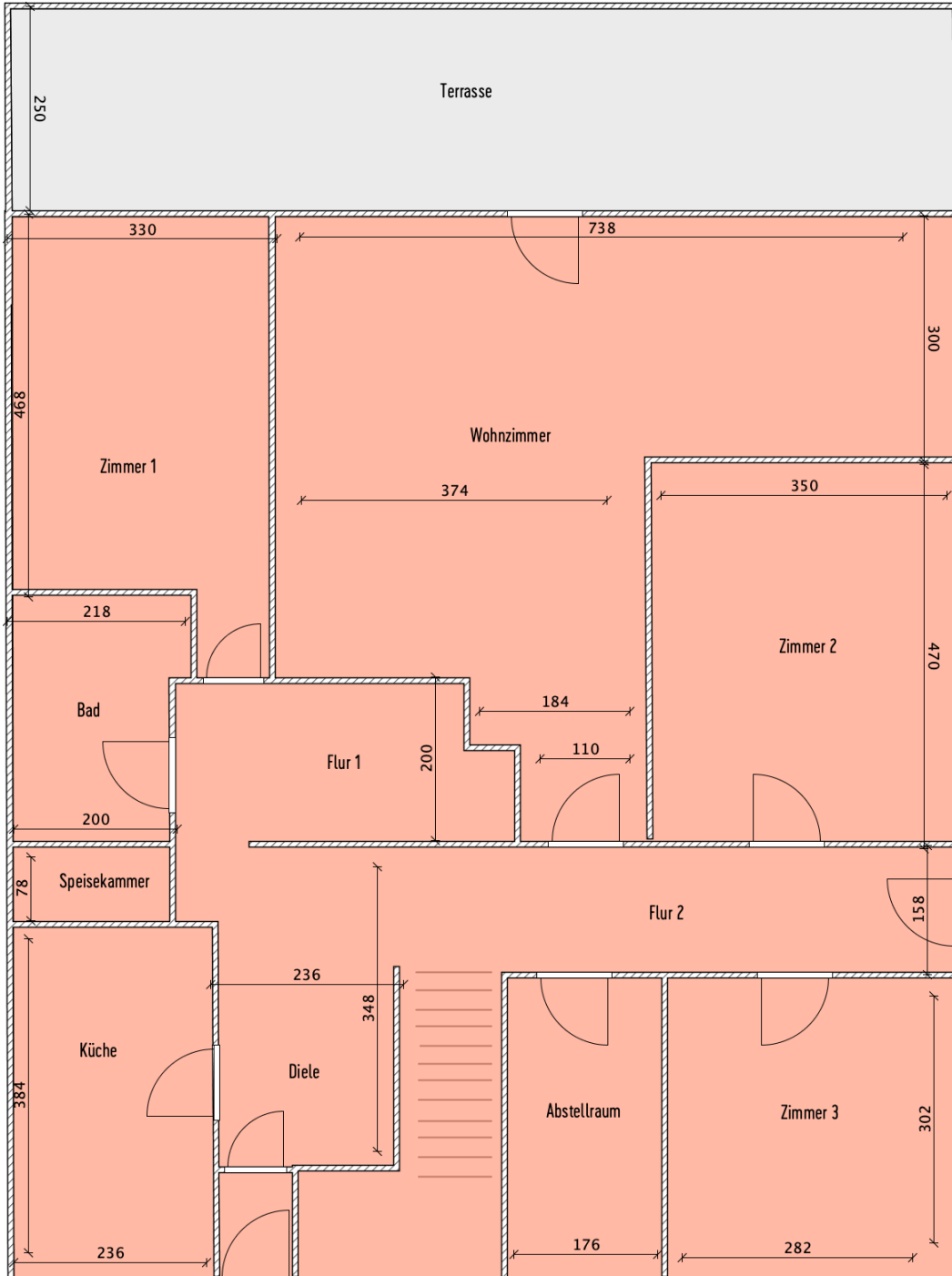
Untergeschoss, Bemaßung in cm
